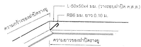
ขยายเหล็กมุมฝาดัดรางยู ค.ส.ล. SCALE NTS
