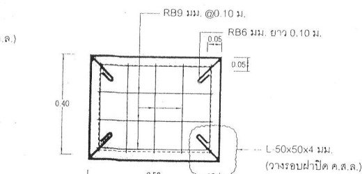
แปลนเสริมเหล็กราง ยู SCALE NTS
