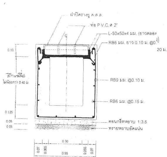
รูปตัด 1 SCALE NTS
