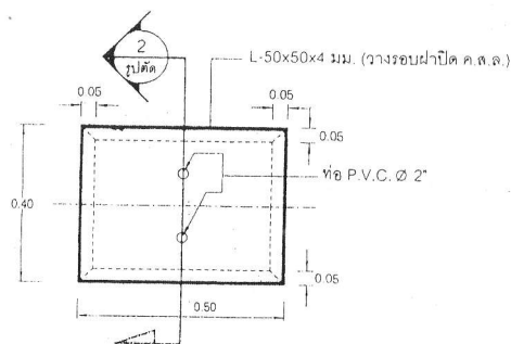
ขยายฝาดัดราง ยู SCALE NTS
