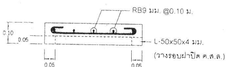
รูปตัด 2 SCALE NTS
