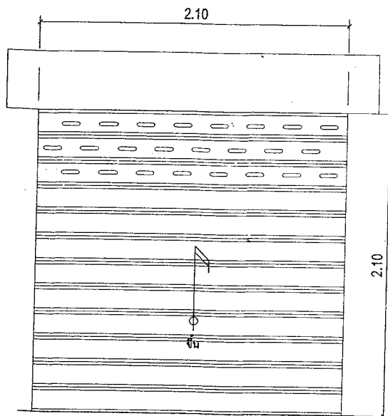
ประตูเหล็กม้วน แบบมีช่องระบายอากาศด้านบน ทำสีกันสนิม พร้อมอุปกรณ์ครบชุด
