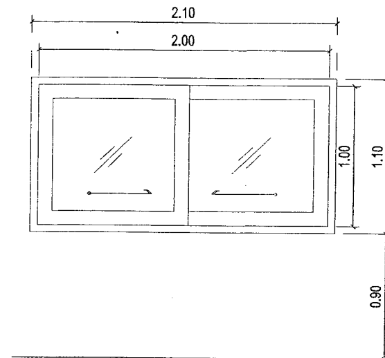
หน้าต่างบานเลื่อนอะลูมิเนียม วงกบอะลูมิเนียม 2x4" สีดำ กรอบบานอะลูมิเนียม 1/2" x 3" สีดำ ลูกพับและช่องมสกรงกระจกเขียวใสหนา 5 มม. พร้อมชุดเหล็กดัดและอุปกรณ์ครบชุด
