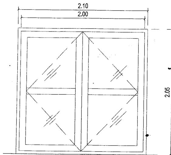
ประตูบานพับคู่อะลูมิเนียม วงกบอะลูมิเนียม 2x4" สีดำ กรอบบานอะลูมิเนียม 1/2" x 3" สีดำ ลูกพับและช่องมสกรงกระจกเขียวใสหนา 5 มม. และอุปกรณ์ครบชุด
