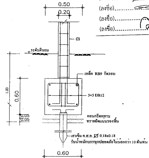
ฐานราก F2
