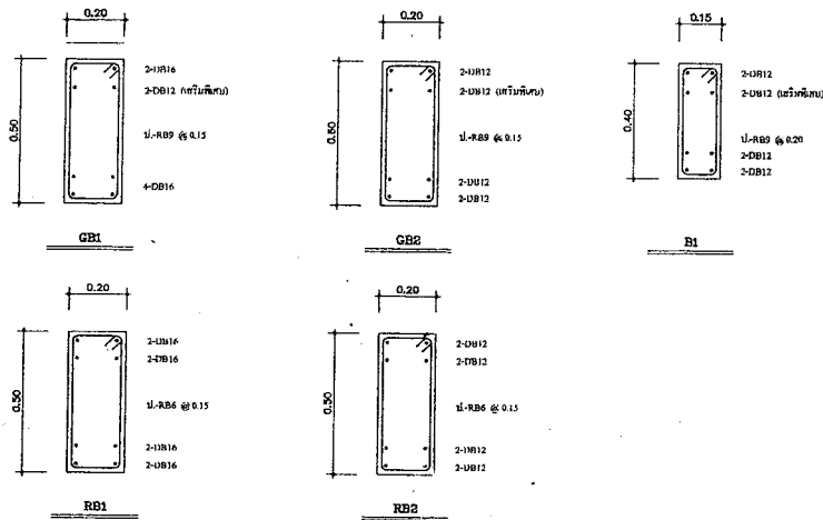
แบบขยายเสริมเหล็กคาน
