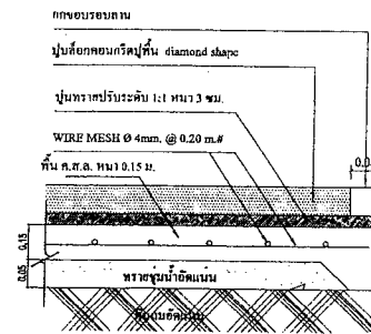
ขยายพื้นล้อยคองกรีต SCALE 1:20
