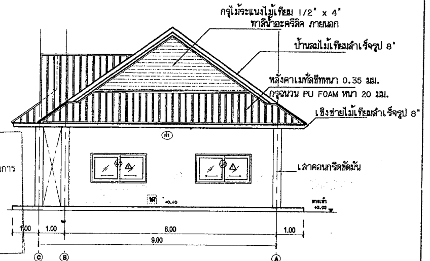
รูปด้าน C ขนาดหน้า 1:100
