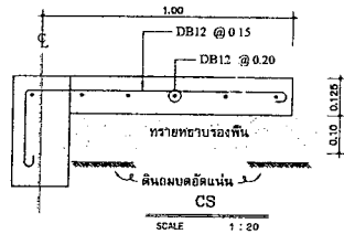
แบบขยายเสริมเหล็กคาน
