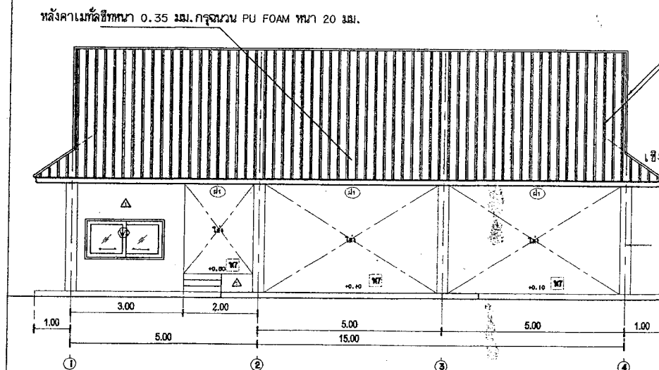
รูปด้าน 8 มาตราส่วน 1:100
