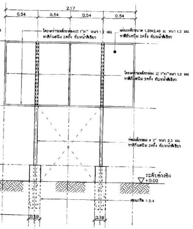
รูปด้านหลัง SCALE 1:20 (ป้ายดาว)
