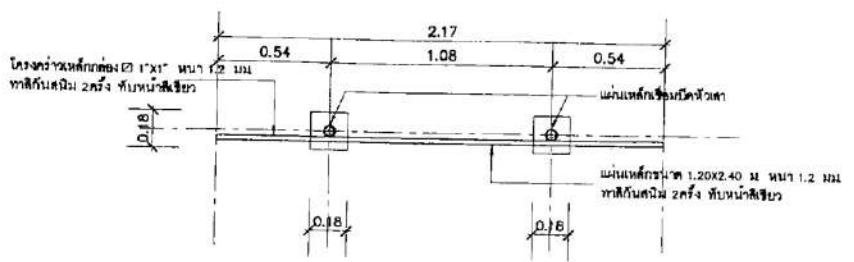
แปลนป้ายโครงการ (ป้ายดาว) SCALE 1:20
