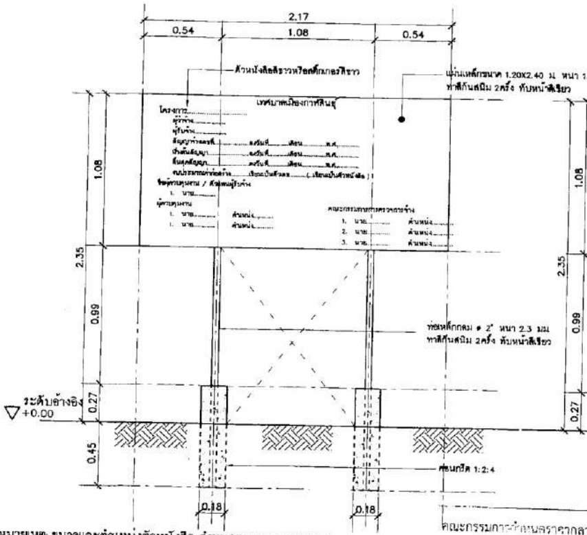
รูปด้านหน้า SCALE 1:20
