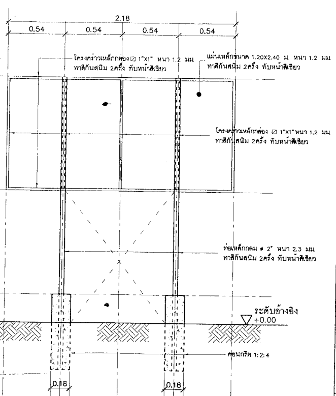
ป้ายประชาสัมพันธ์โครงการ (ป้ายชั่วคราว) SCALE 1:25
