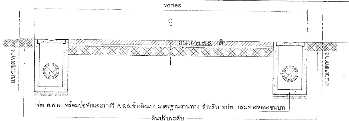
รูปตัด 1 - 1 SCALE NTS.
