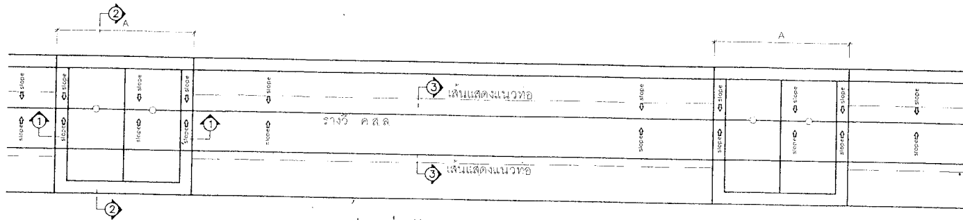
แปลนบ่อดัก และรางวี คสล. (กรณีบนผิวจราจร)
