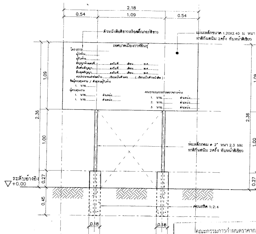
รูปด้านหน้า SCALE 1:25
