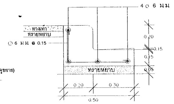
แบบขยายคันหิน (A) SCALE NTS
