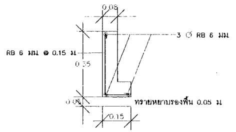
แบบขยายคันหิน (B) SCALE NTS
