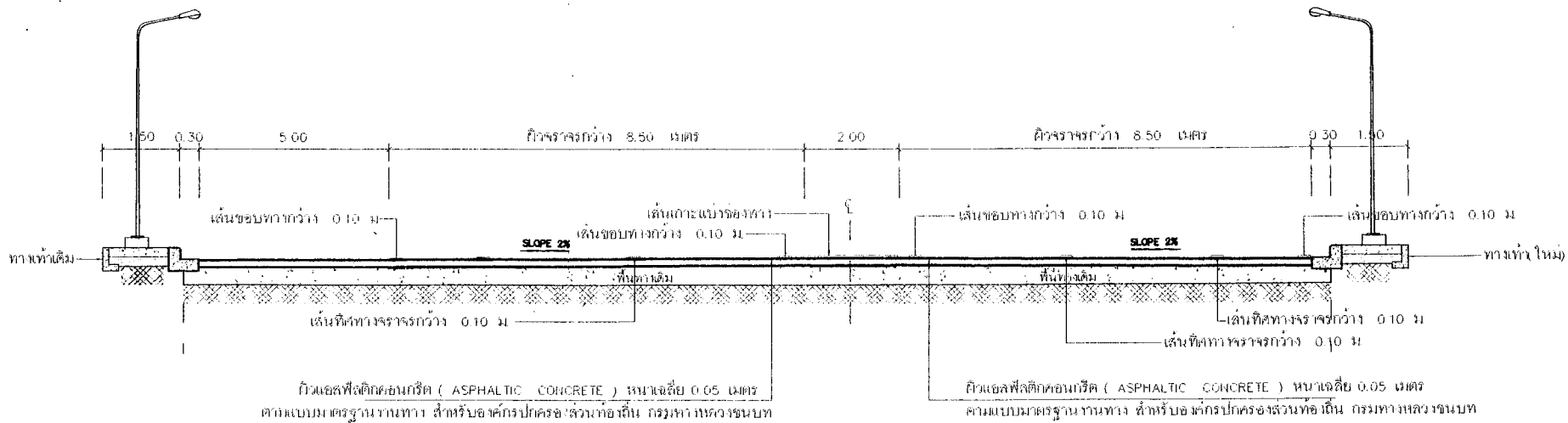
รูปตัด 3-3 SCALE NTS.
