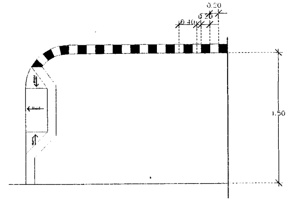
แบบขยายลัดทางเท้าแบบ A SCALE NTS
