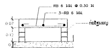
แบบขยายช่องรับน้ำ SCALE NTS
