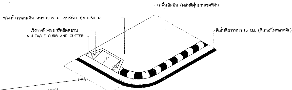
แบบขยายทางเท้าแบบ A SCALE NTS
