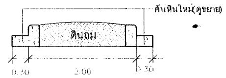
แบบขยายเกาะกลาง SCALE NTS
