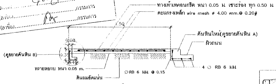
รูปตัดทางเท้าแบบ A SCALE NTS
