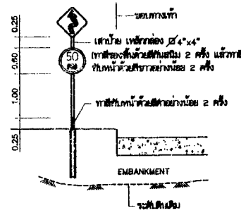
การปักเสาป้ายบังคับจราจรบนป้ายเตือน
