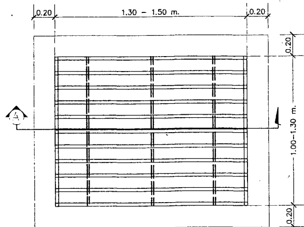
ฝาบ่อพักเหล็กตะแกรง มาตราส่วน NTS.
