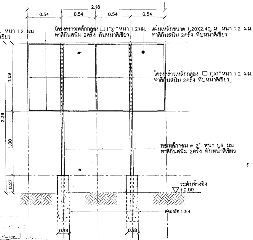
รูปด้านหลัง (ป้ายถาวร) SCALE 1:25
