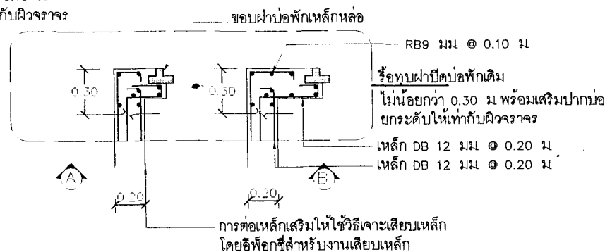
ขยายเสริมปากบ่อพัก แบบฝาบ่อพักเหล็กหล่อ มาตราส่วน NTS.
