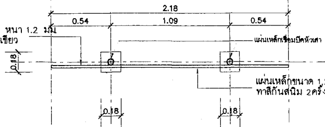
แปลนป้ายโครงการ (ป้ายถาวร) SCALE 1:25
