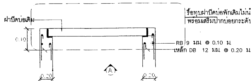
ฝาบ่อพักเหล็กตะแกรง มาตราส่วน NTS.
