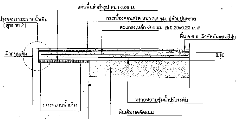
รูปตัด Y มาตราส่วน 1:25
