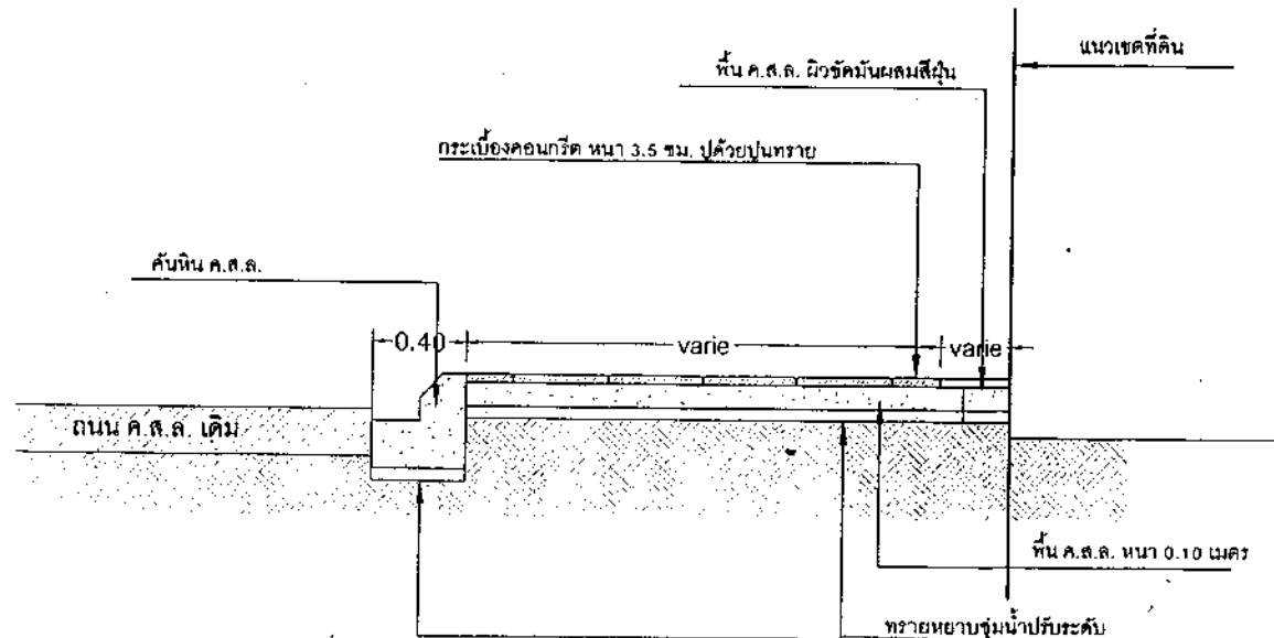
รูปตัด X
