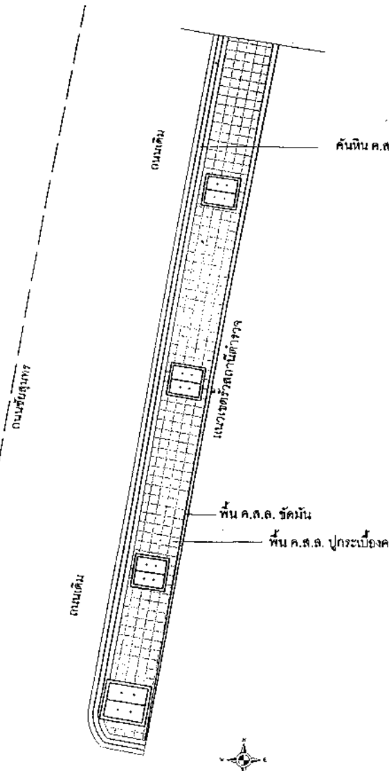
แปลนทางเท้า 83-1 มาตราส่วน 1:150 (ดูขยายทางเท้าแบบที่ 2)
