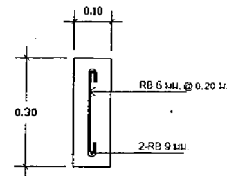
ขยายคันทัน มาตราส่วน 1:10
