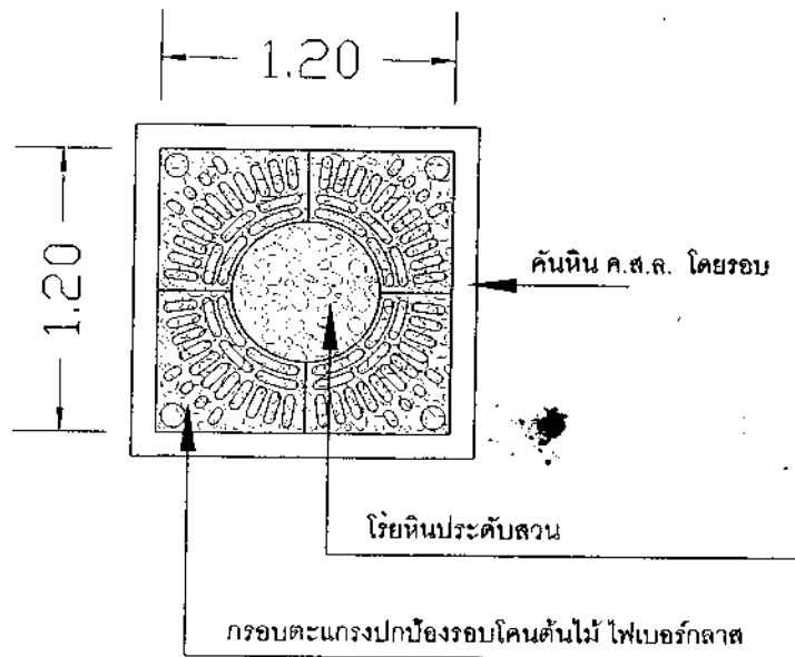
แปลนกรอบตะแกรงปกป้องรอบโคนต้นไม้ มาตราส่วน 1:25
