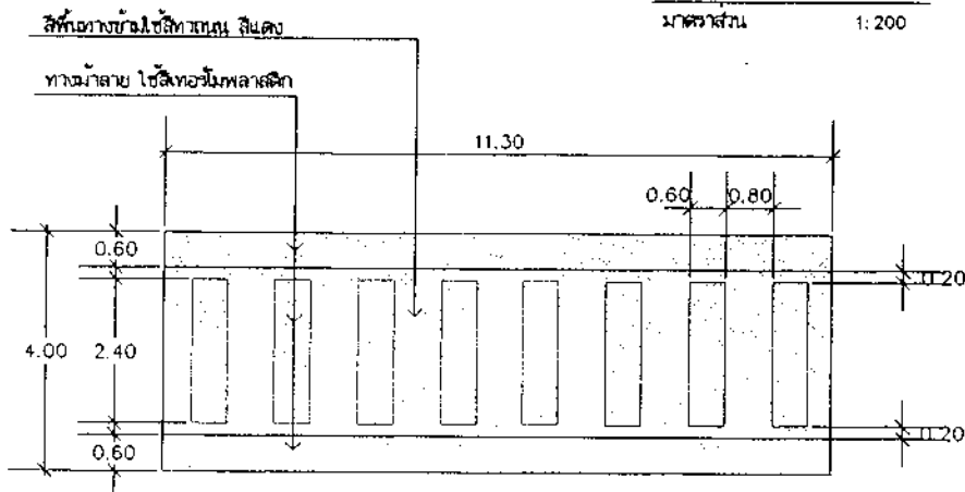
แปลนทางข้าม
