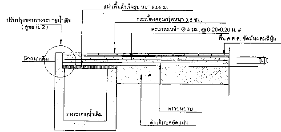
รูปตัด Y มาตราส่วน 1:25
