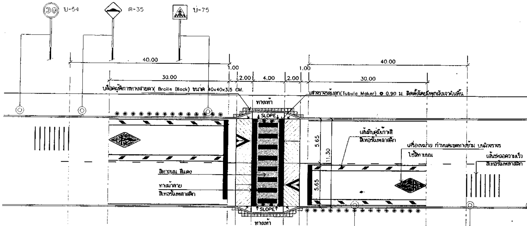
แปลนทางข้าม
