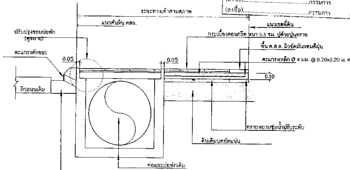
รูปตัด Y
