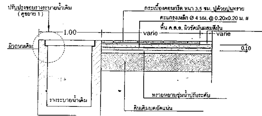
รูปตัด X มาตราส่วน 1:25
