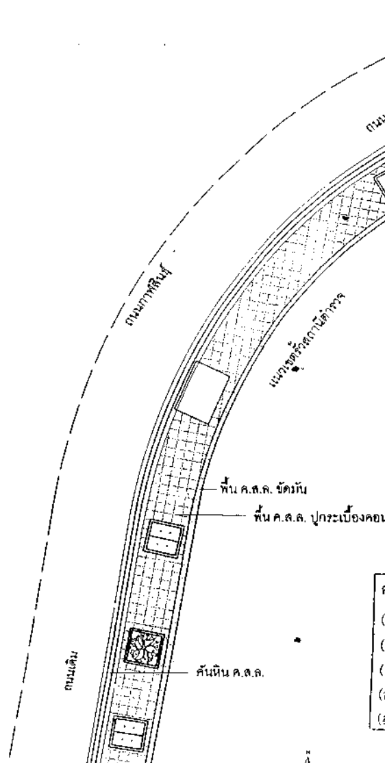
แปลนทางเท้า 83-2 มาตราส่วน 1:150 (ดูขยายทางเท้าแบบที่ 2)
