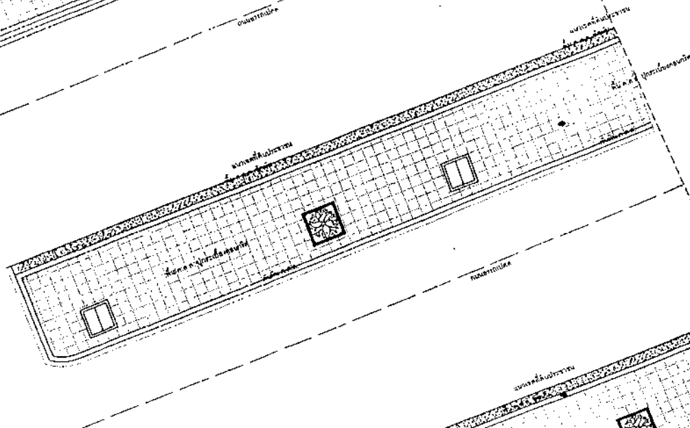
แปลนทางเท้า 46-1 มาตราส่วน 1:150 (ดูขยายทางเท้าแบบที่ 2)
